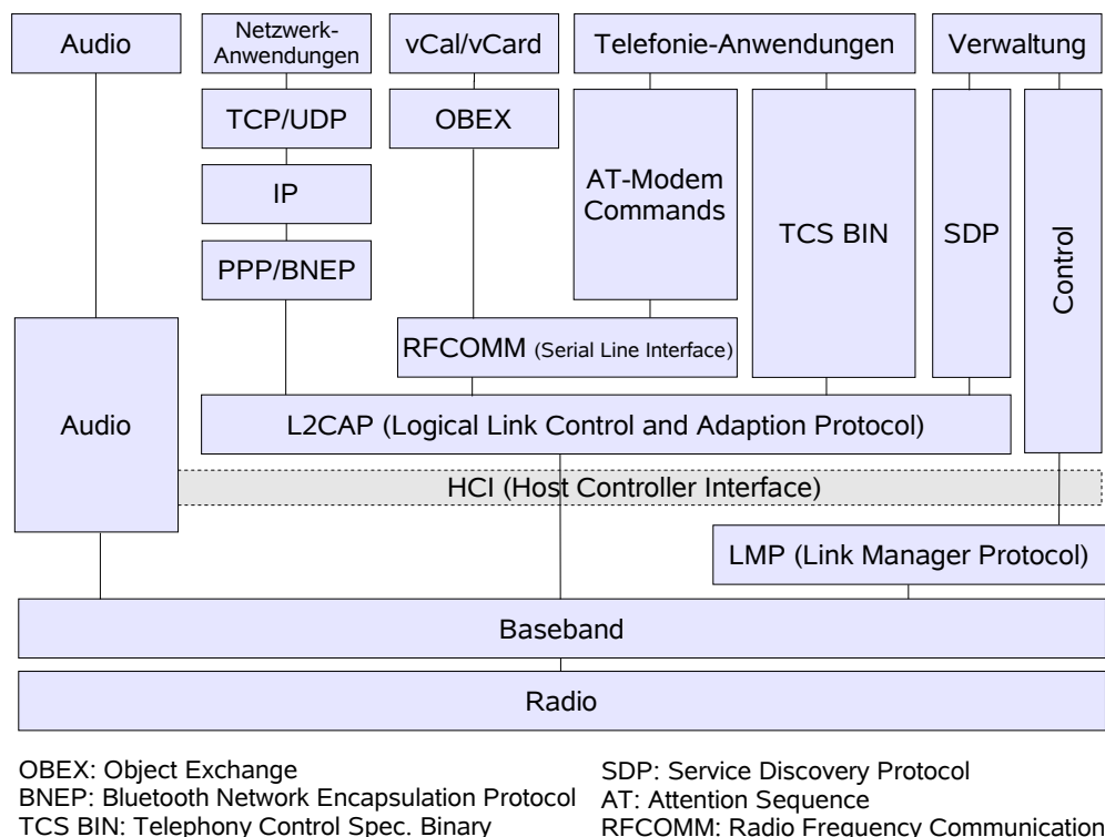
Abbildung 3: Bluetooth-Protokollstapel
